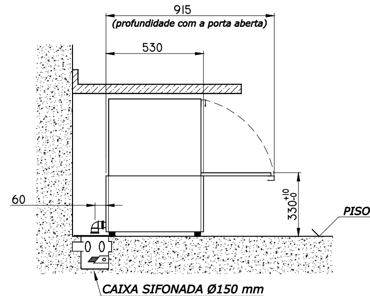
VISTA LATERAL
