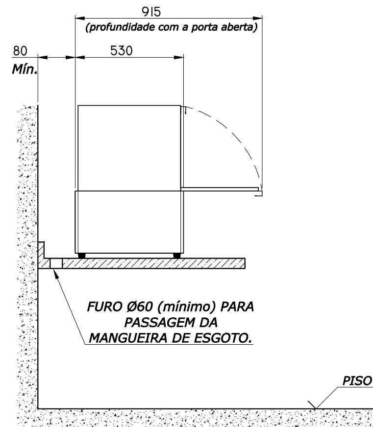
VISTA LATERAL
