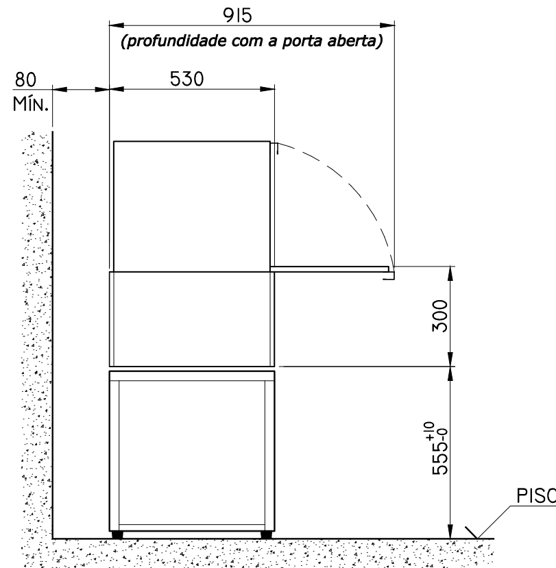
VISTA LATERAL
